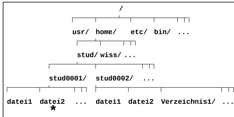
Abbildung 2.1: Unix-Verzeichnisbaum
