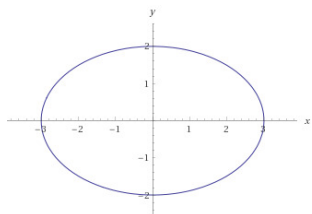
Ellipse mit Hauptachsen a = 3 und b = 2 , Wolfram Alpha
